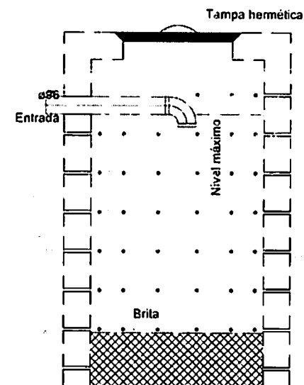
Sumidouro - Pavimento Corte 1 - ESC. 1:25
