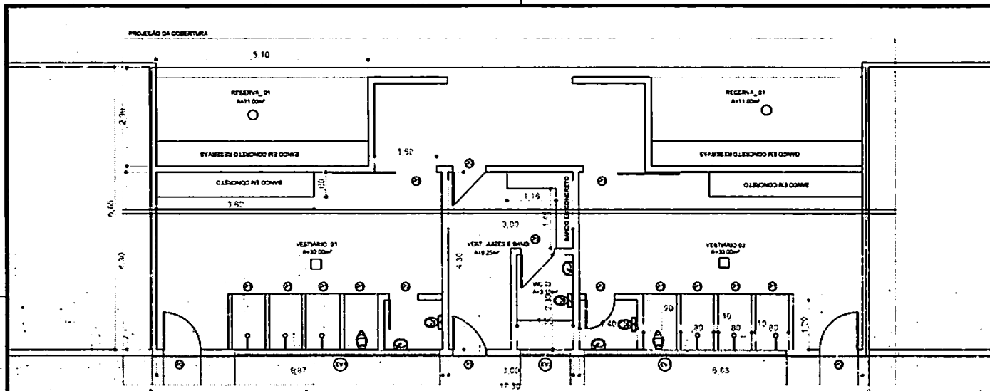
01 REFORMA DE CAMPO DE FUTEBOL VESTIÁRIO ESC. 1:100
