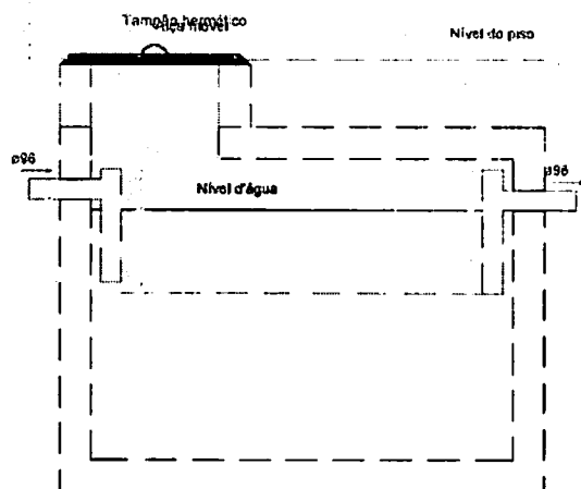
Tanque séptico - Pavimento Corte 1 - ESC. 1:25
