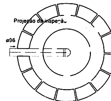
Sumidouro - Pavimento Planta baixa - ESC. 1:25
