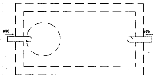
Tanque séptico - Pavimento Planta baixa - ESC. 1:25
