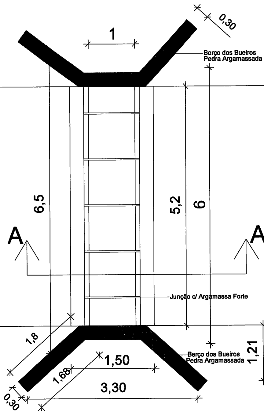
PLANTA BAIXA CORPO DE BSTC 1,00M
